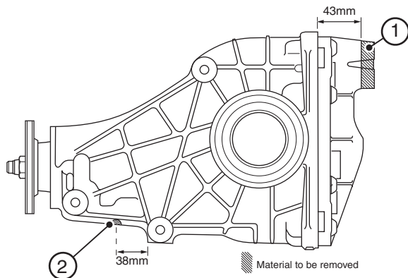
1 Rear lug 2 Underside
